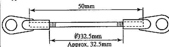
X型レバー / エルロンレバーロッド (2セット) X-type lever / Aileron lever rod (2 sets)
