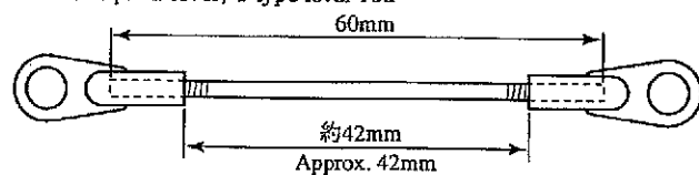
コレクティブピッチロッド (2セット)
