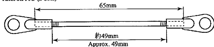
エルロンロッド (2セット) Aileron rod (2 sets)
