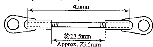
コレクティブピッチロッド (2セット)
