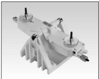
1077 ROTORBLATTWAAGE
