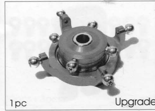
HS1062 Aluminum swashplate(V2)
