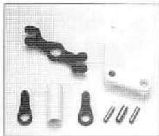
テールピッチレバ ーセット (SR) No.H3123 ●700 Tail Pitch Lever Set (SR)
