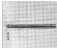
テールアウトプット シャフト No.H3043 ●700 Tail Output Shaft
