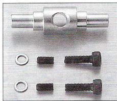
H6053R テールセンターハブ ¥800
