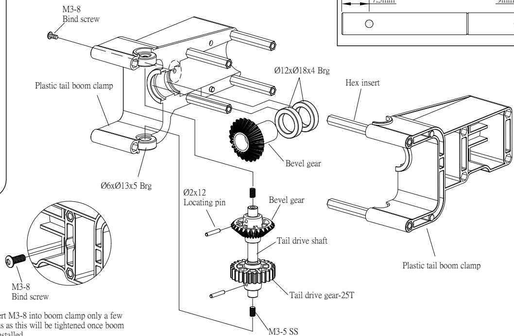
M3-5 SS
